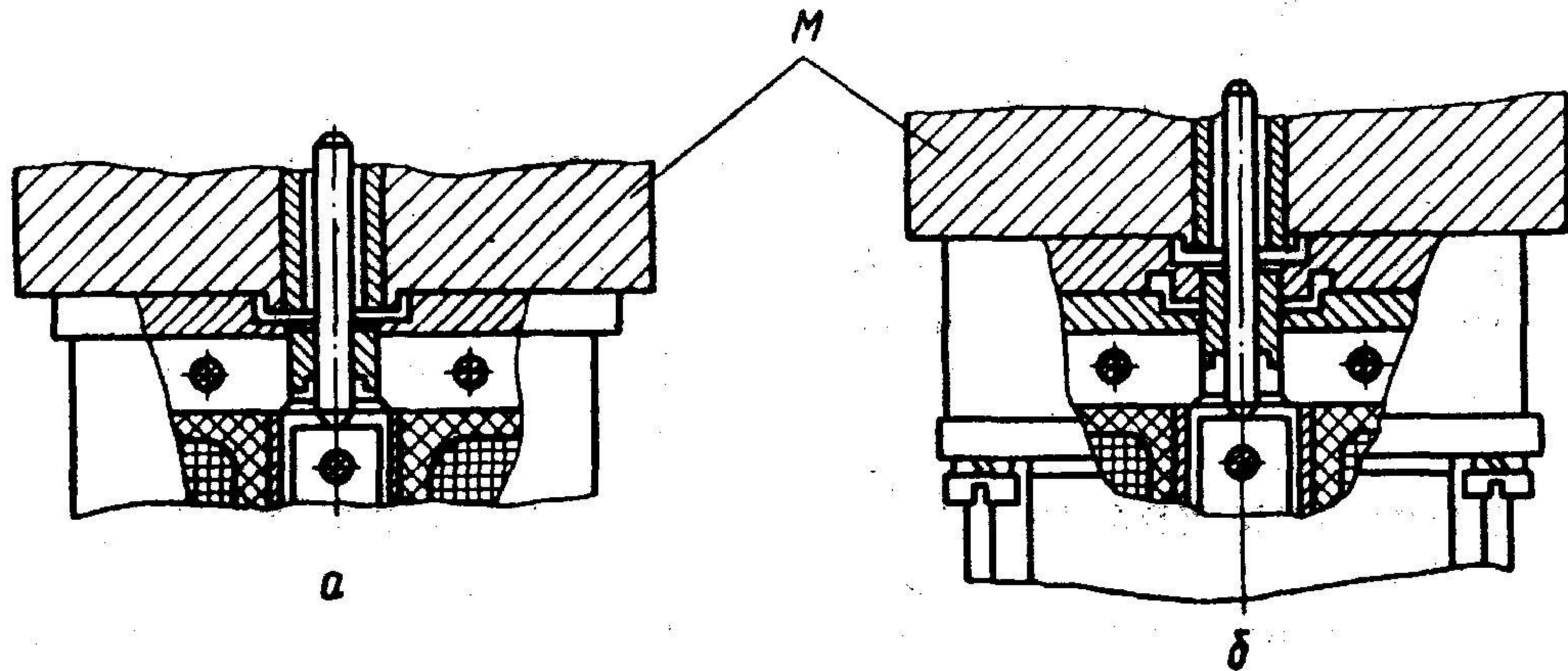
Рис. 4. a — открытое и защищенное исполнение; б — пылезащищенное исполнение; М — исполнительный механизм
