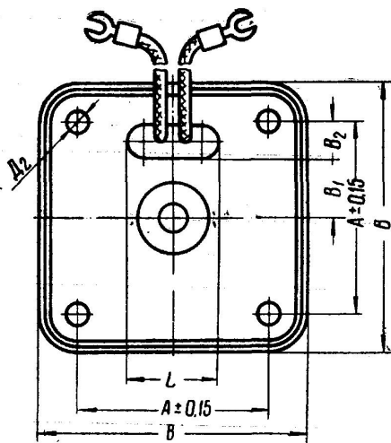
Рис. 2. Габаритные и установочные размеры толкающих электромагнитов серии МТ защищенного исполнения: С — ход якоря
